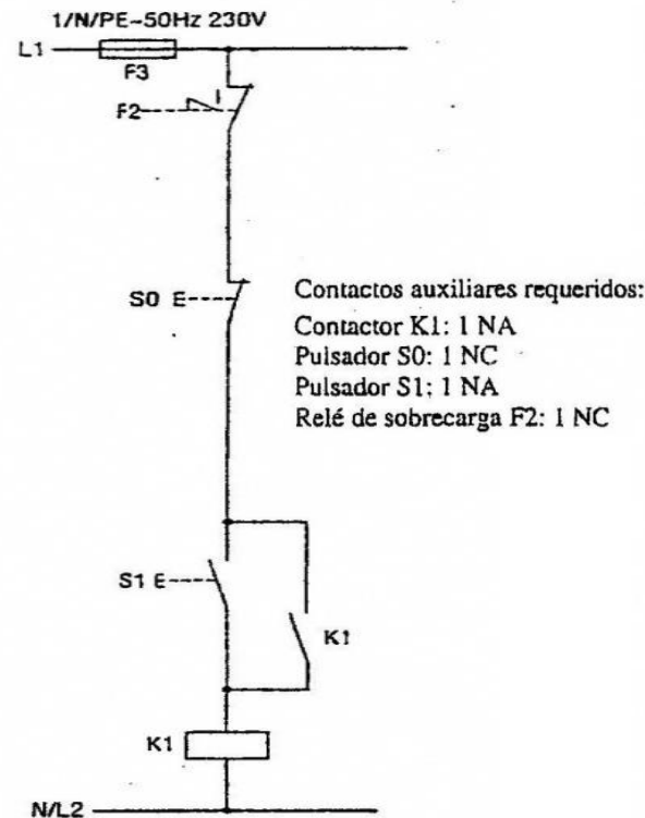
b) Circuito auxiliar para operación por pulsador
